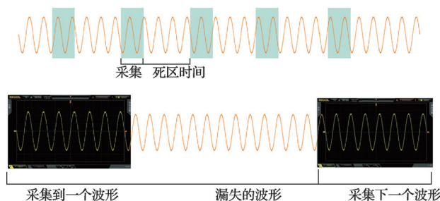
图1 波形捕获示意
