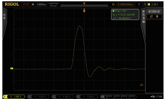
图7 停止录制
