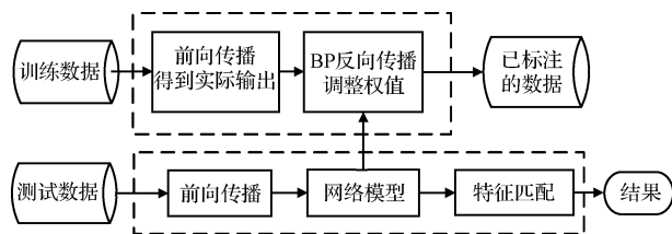
图 2 CNN 的处理流程
