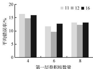
图11 不同卷积核数量对错误率的影响
