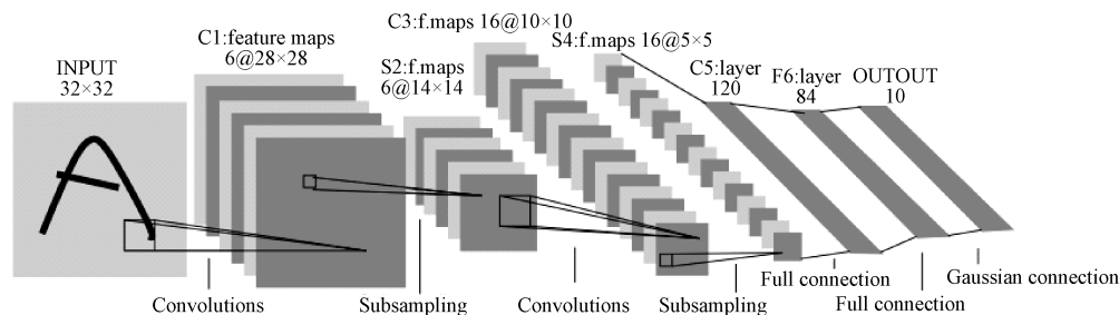
图 1 LeNet-5 结构
