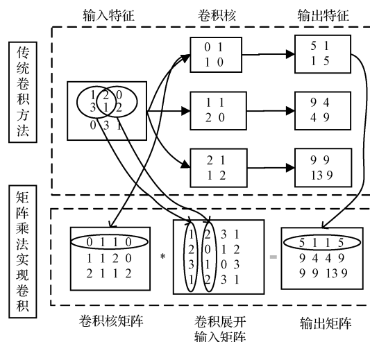
图 6 卷积展开例子
