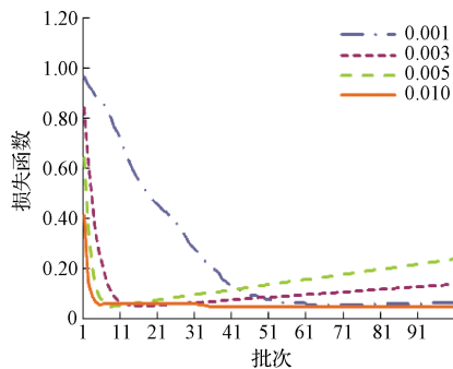
图 8 不同学习率对损失函数的影响
