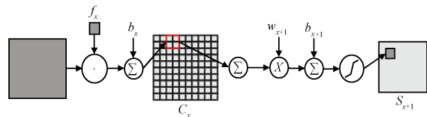
图 3 卷积和子采样过程
