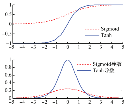
图 4 Sigmoid 函数、tanh 函数及其导数曲线
