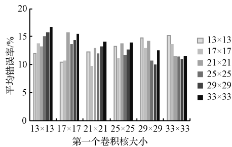
图 10 不同卷积核对识别错误率的影响
